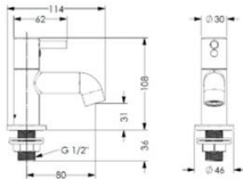
Peg Lever Tap
